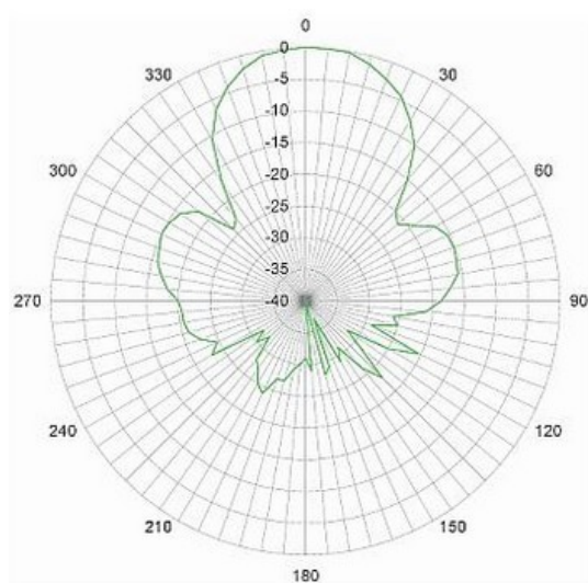
H-Plane
